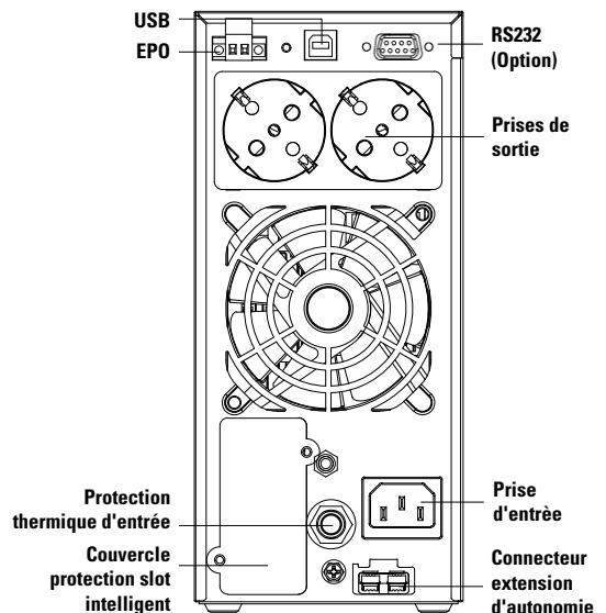
Modèle de 0,7 à 1 kVA -B1-
