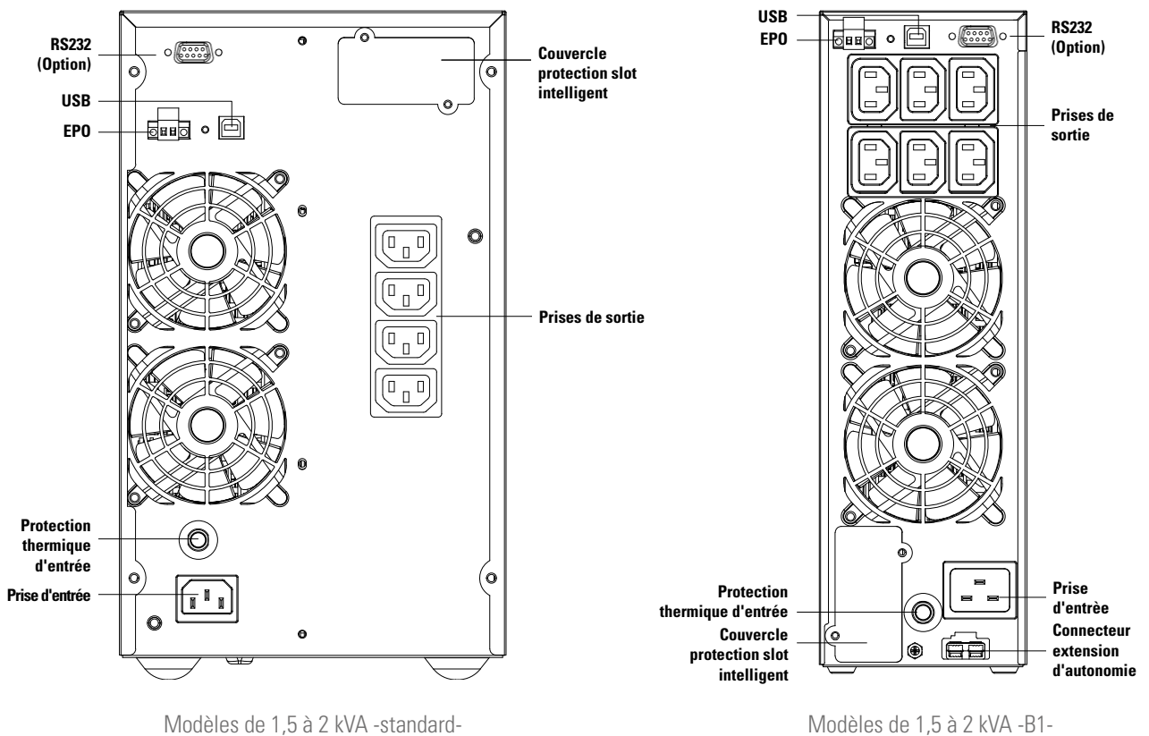
Fig. 4. Vue arrière, modèles de 1,5 à 2 kVA avec connecteurs de sortie IEC
