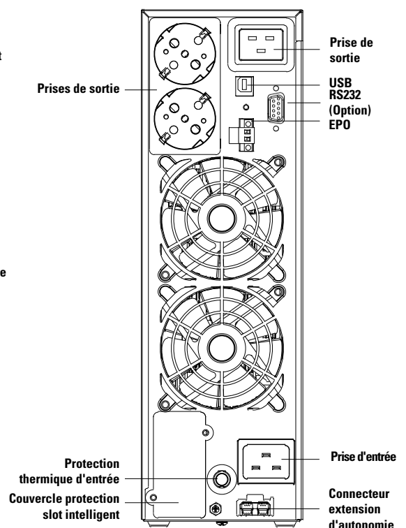
Modèle de 3 kVA -B1-
