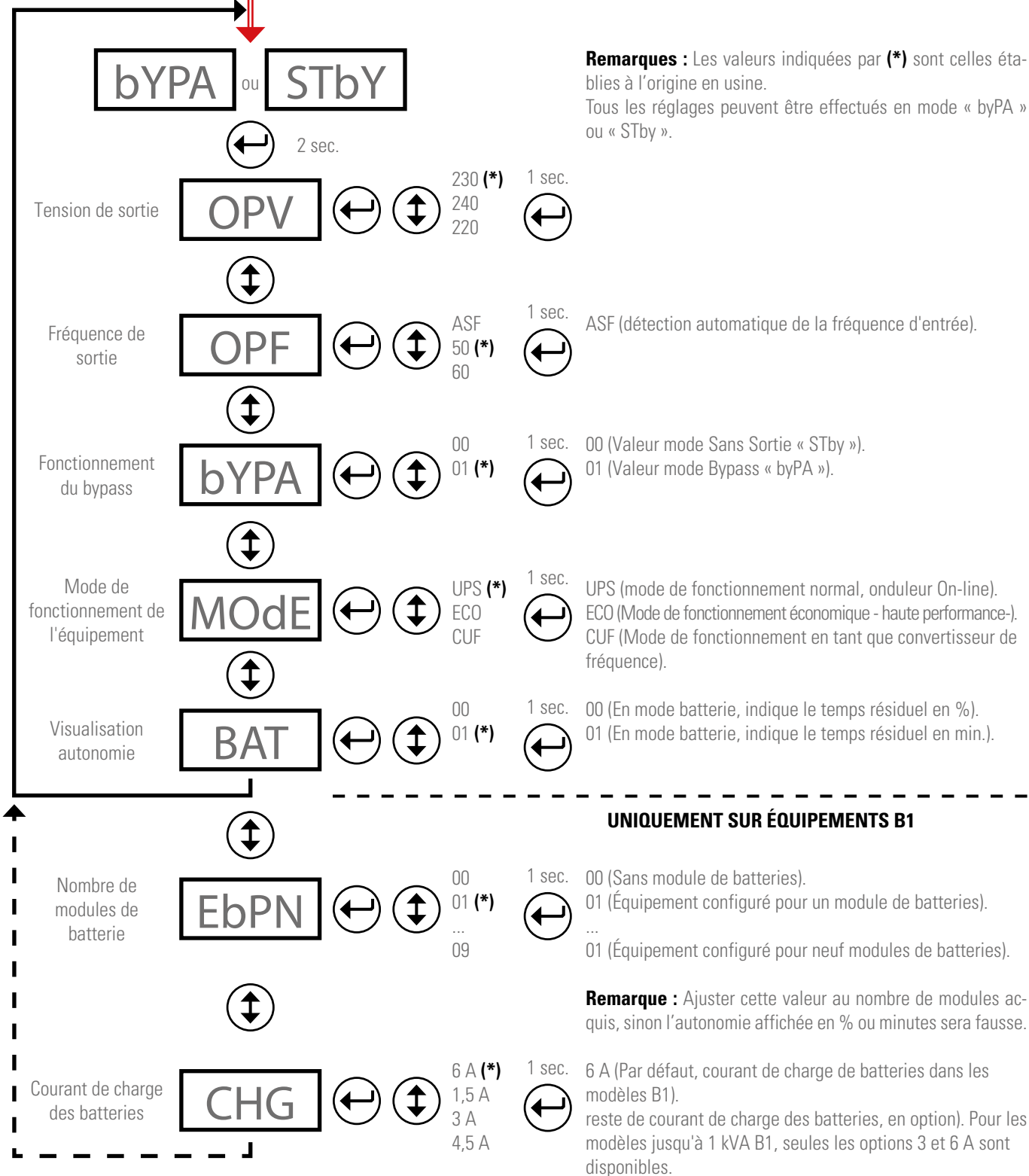
Fig. 20. Carte des écrans de réglage.
