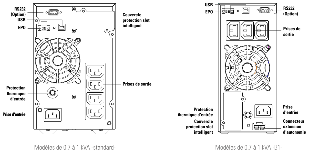
Fig. 3. Vue arrière, modèles de 0,7 à 1 kVA avec connecteurs de sortie IEC.
