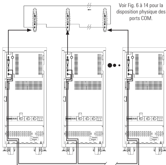
Fig. 38. Connexion du BUS de communication.
