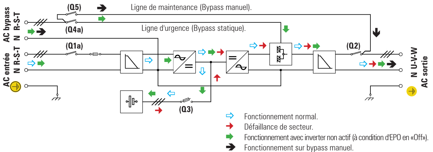
Fig. 26. Schéma de blocs ONDULEUR SLC CUBE3+ B avec de flux de fonctionnement.
