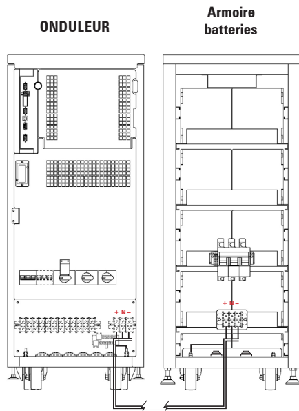
Fig. 33. Connexion entre ONDULEUR et des armoires de batteries.
