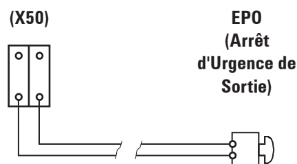
Fig. 37. Bornes de connexion pour interrupteur ou bouton externe d'arrêt d'urgence (EPO), propriété de l'utilisateur.
