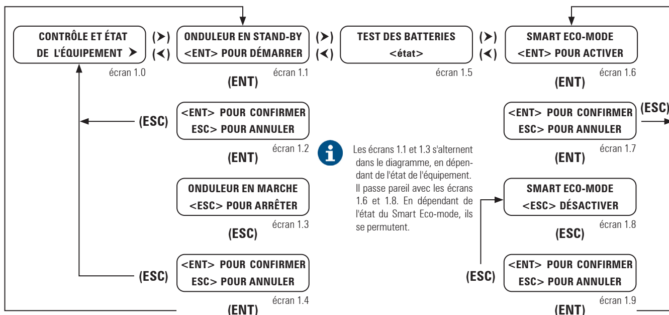
Fig. 49. Sous-menu d'écrans 1.0. Mise en marche / arrêt.
