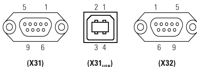
Fig. 36. Connecteur DB9 ( X31 ) et ( X32 ), et ( X31 USB ).
