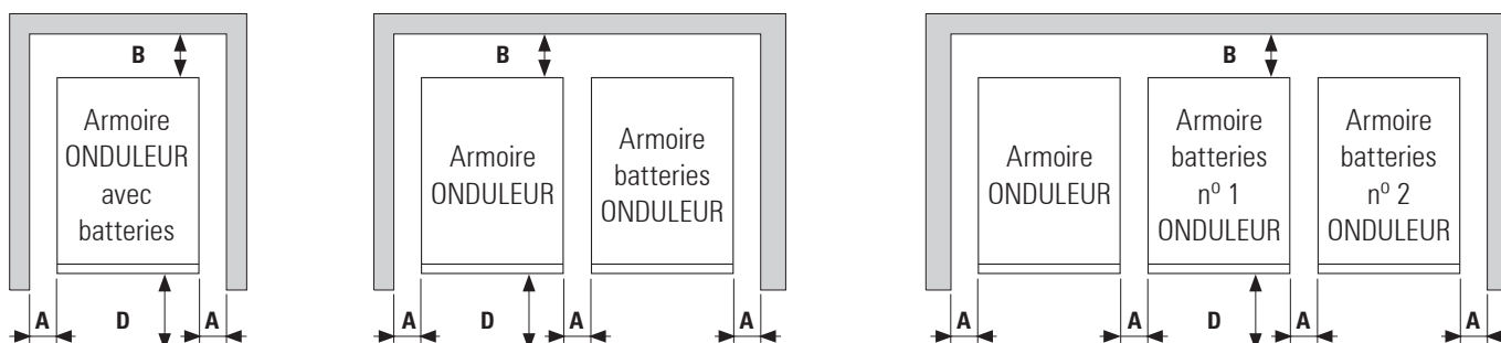
Fig. 30. Dimensions minimales périphériques pour la ventilation de l'ONDULEUR.
