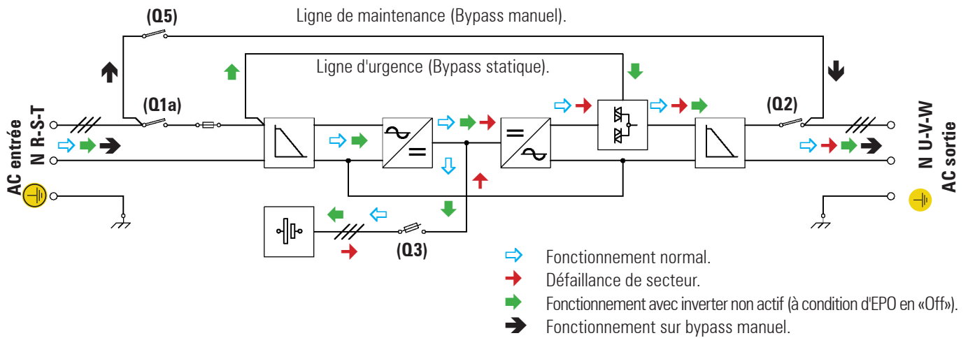
Fig. 25. Schéma de blocs ONDULEUR SLC CUBE3+ avec de flux de fonctionnement.
