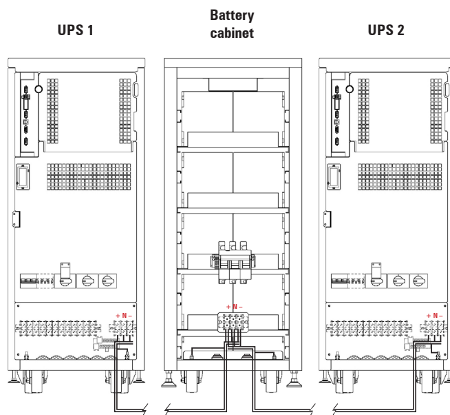
Fig. 35. Exemple de connexion de deux ONDULEURS en parallèle avec un groupe de batteries commun.
