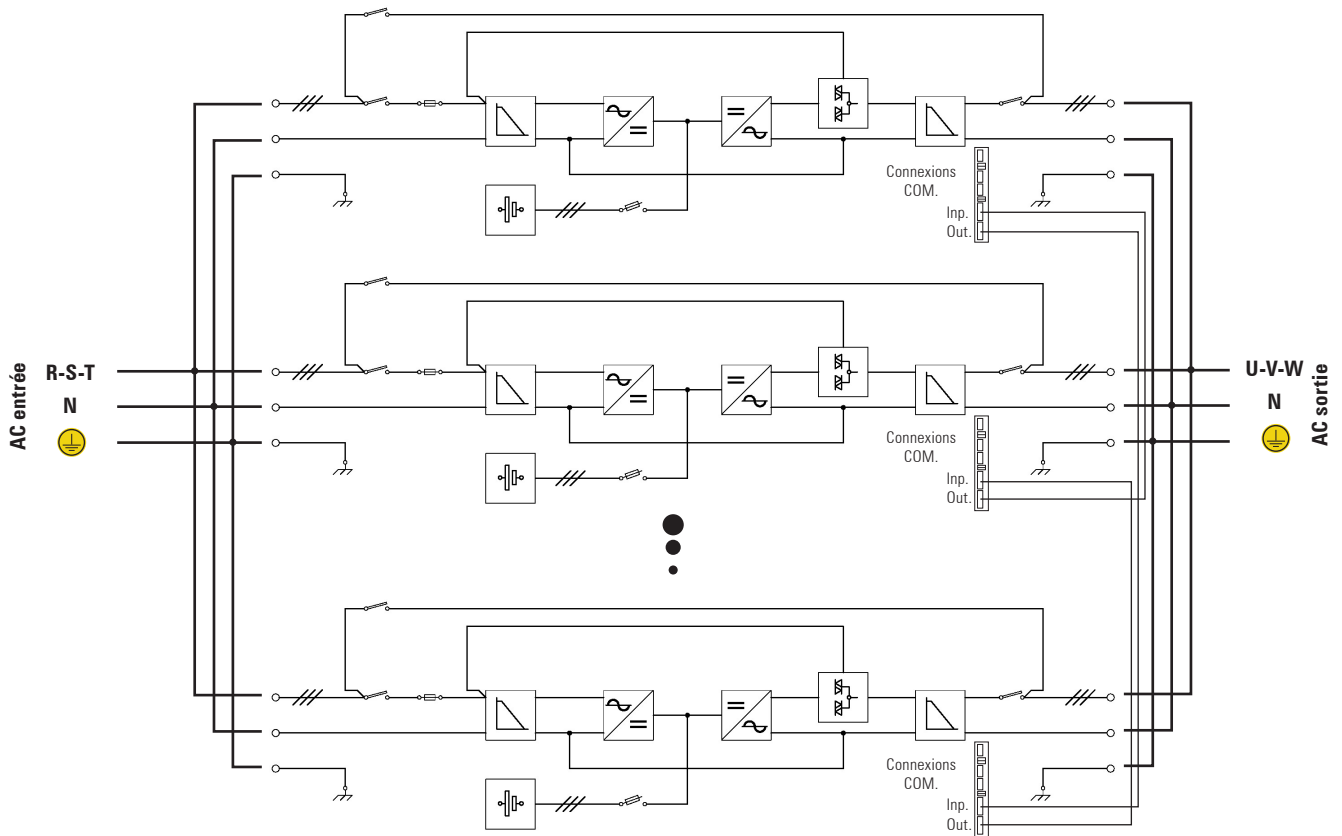
Fig. 27. Schémade blocs, connexions système en parallèle jusqu'à 4 équipements SLC CUBE3+ .
