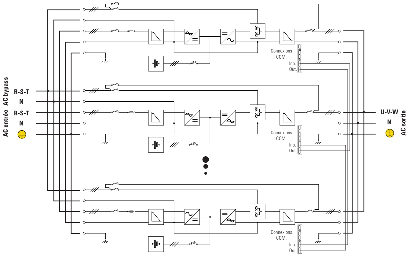
Fig. 28. Schéma de blocs, connexion système en parallèle jusqu'à 4 équipements SLC CUBE3+ B .
