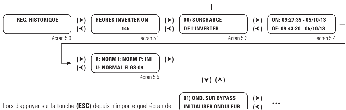
Fig. 53. Écran 5.0 «Historique» et ses sous-menus.
