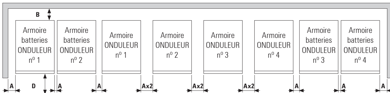
Fig. 31. Dimensions minimales périphériques pour la ventilation d'un système.
