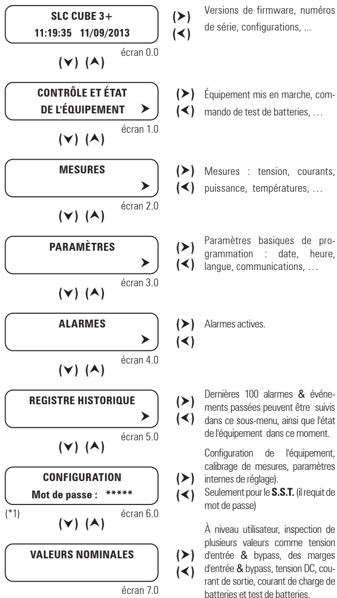
Fig. 47. Classification des menus et sous-menus montrés sur le LCD.
