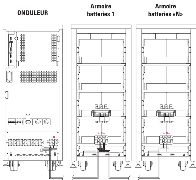
Fig. 34. Exemple de connexion entre ONDULEUR et deux armoires de batteries.
