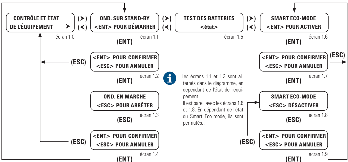
Fig. 43. Diagramme, procédure de mise en marche / arrêt.
